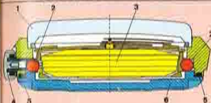
Das schwebende Werk der Certina-DS
